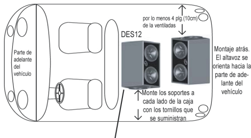
Montaje adelante. El altavoz se orienta hacia la parte de atrás del vehículo
